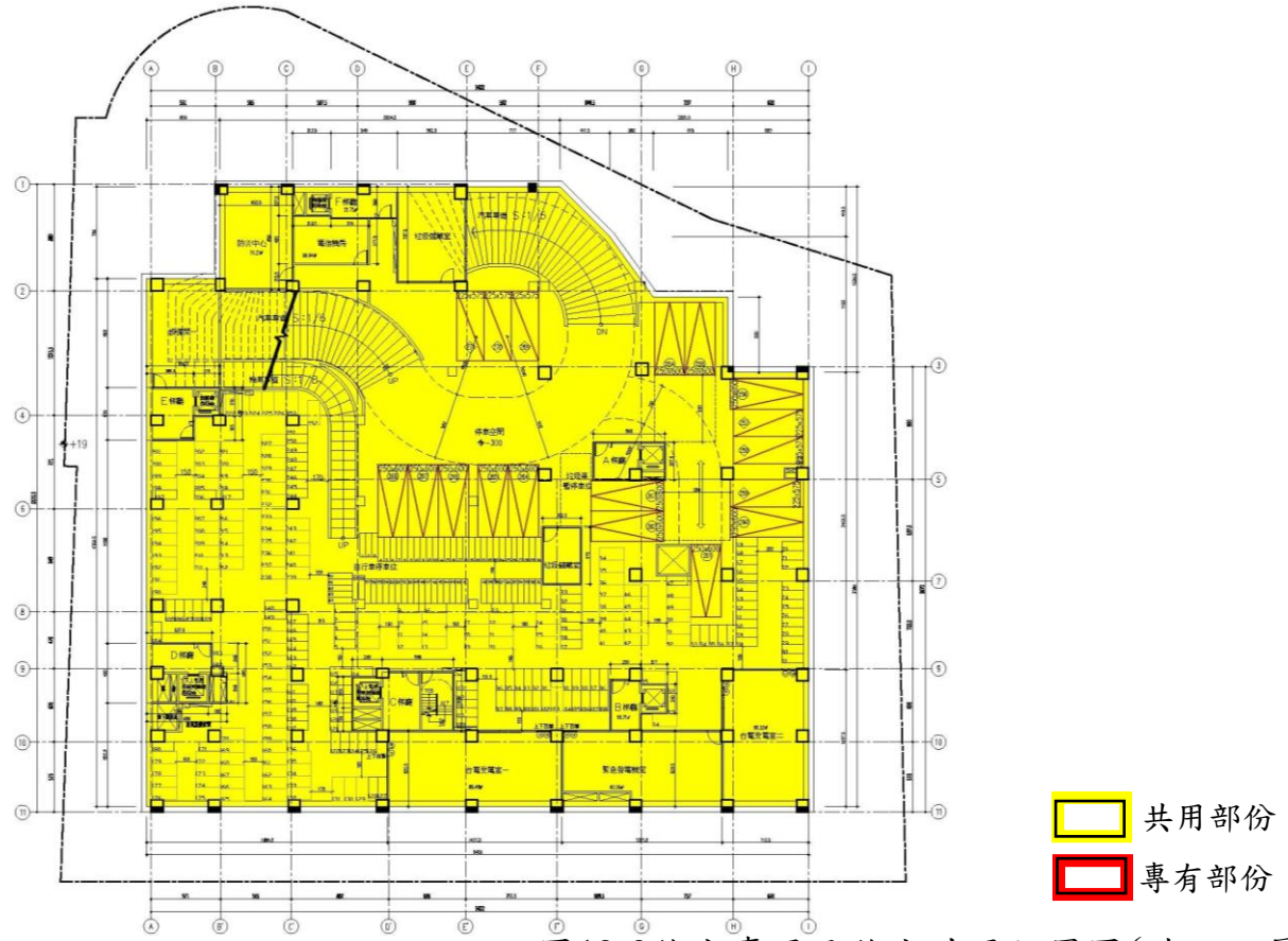
圖19-9約定專用及約定共用位置圖(地下一層)
