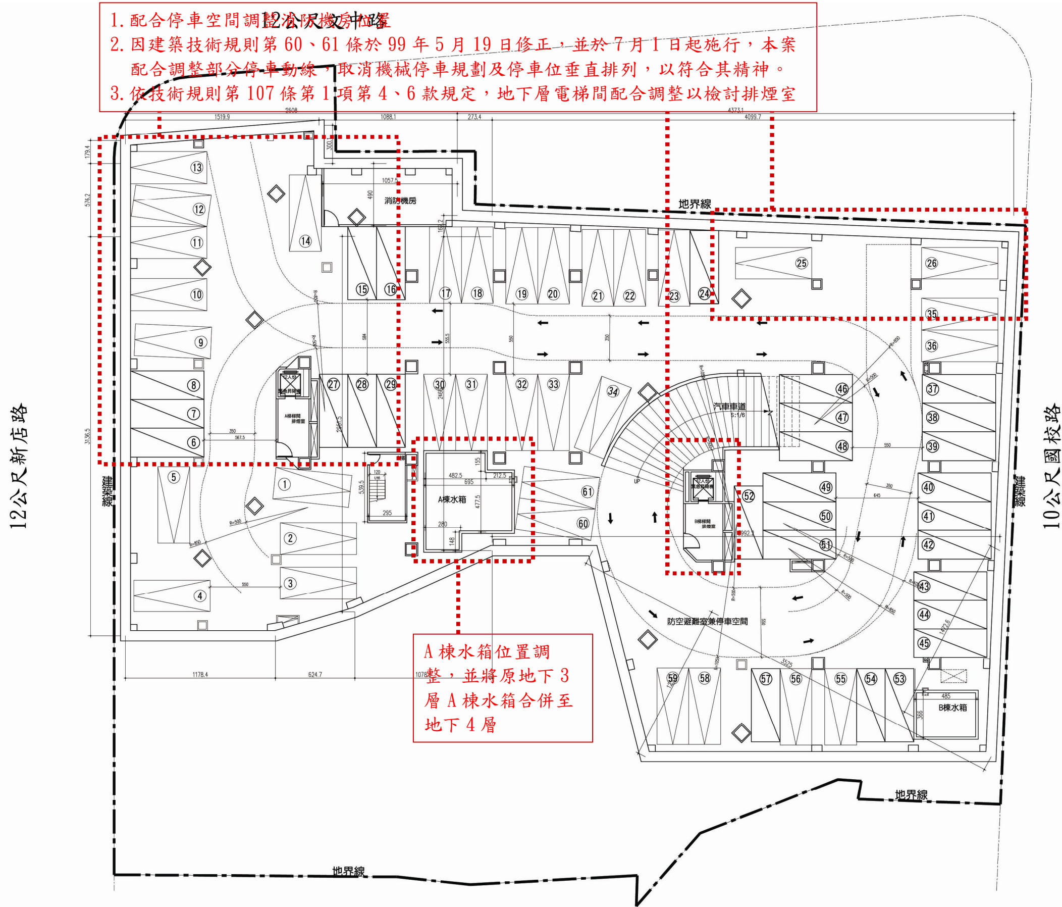
地下四層平面圖 (修正後)
