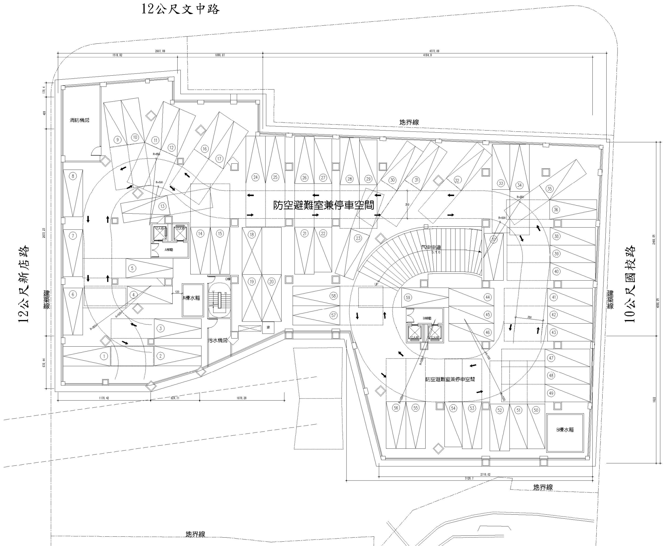
地下四層平面圖 (修正前)
