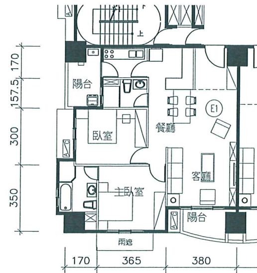
E1戶
