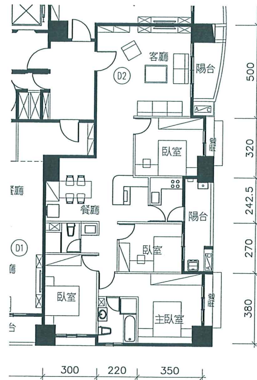
D2戶
