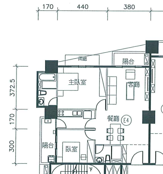
E4戶
