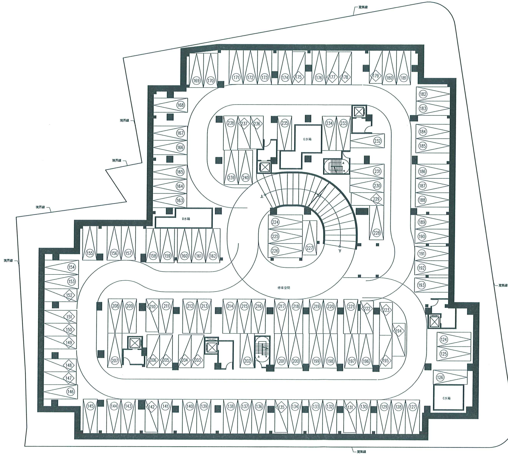
1 A2-2 地下三層平面圖 S:1/400
